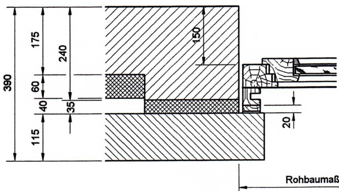
Horizontalschnitt
